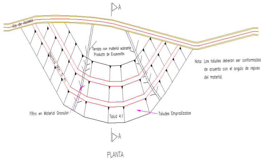
Figura 7-2 ZODME Típico
