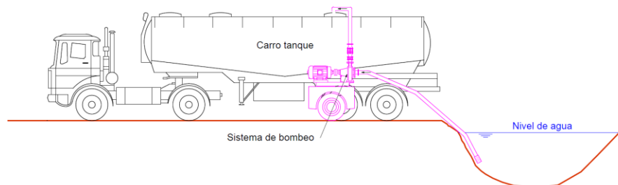
Figura 7-14 Sistema típico de captación
