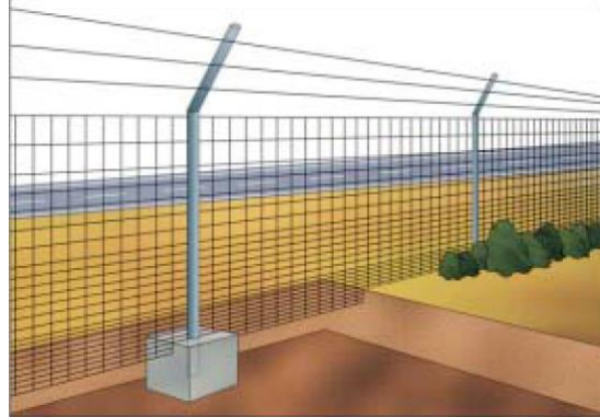
Esquema tipo de cerramiento perimetral
