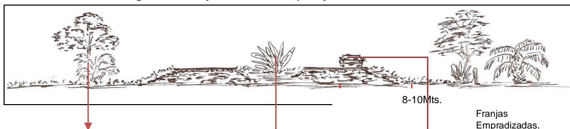
Figura 7-22 Franjas de adecuación paisajística en el derecho de vía
