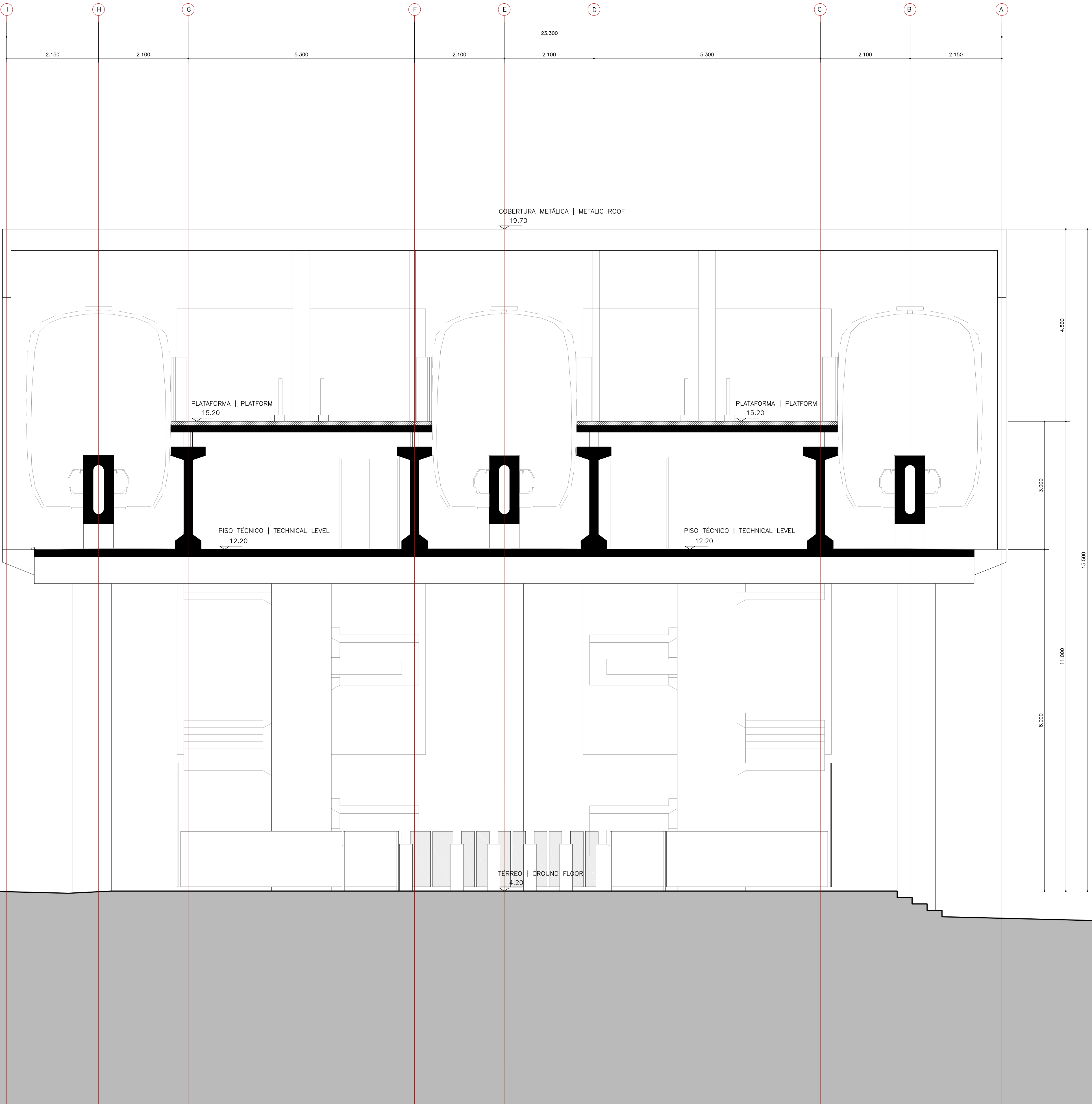
CORTE BB ESCALA | SCALE 1:30
