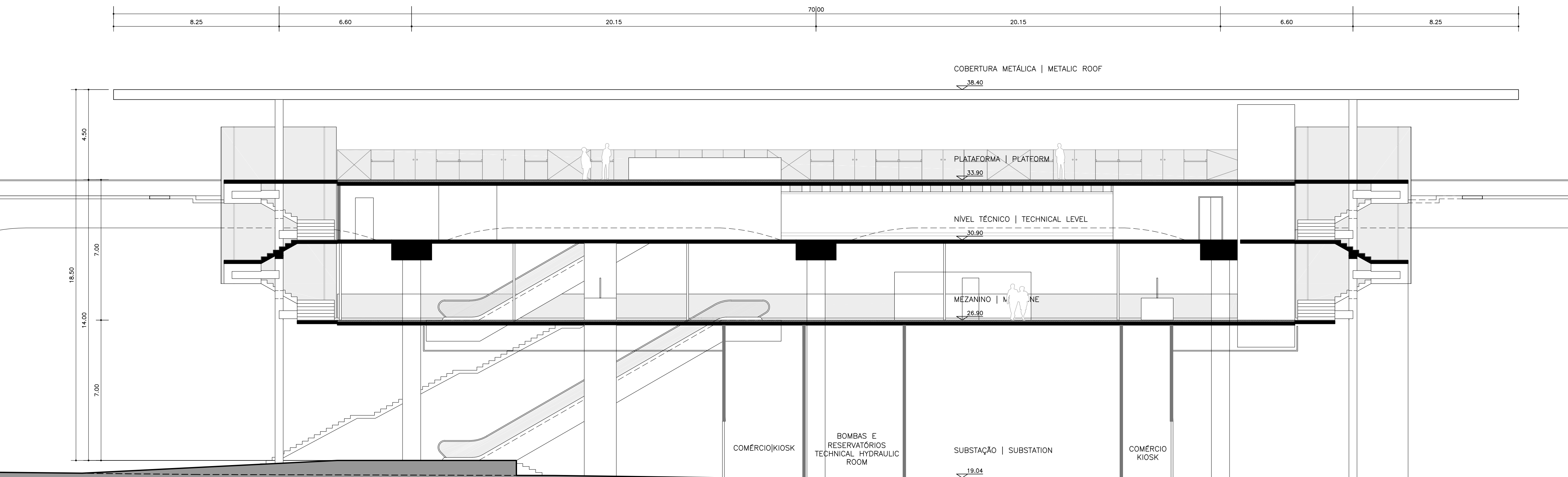
CORTE BB ESCALA | SCALE 1:125
