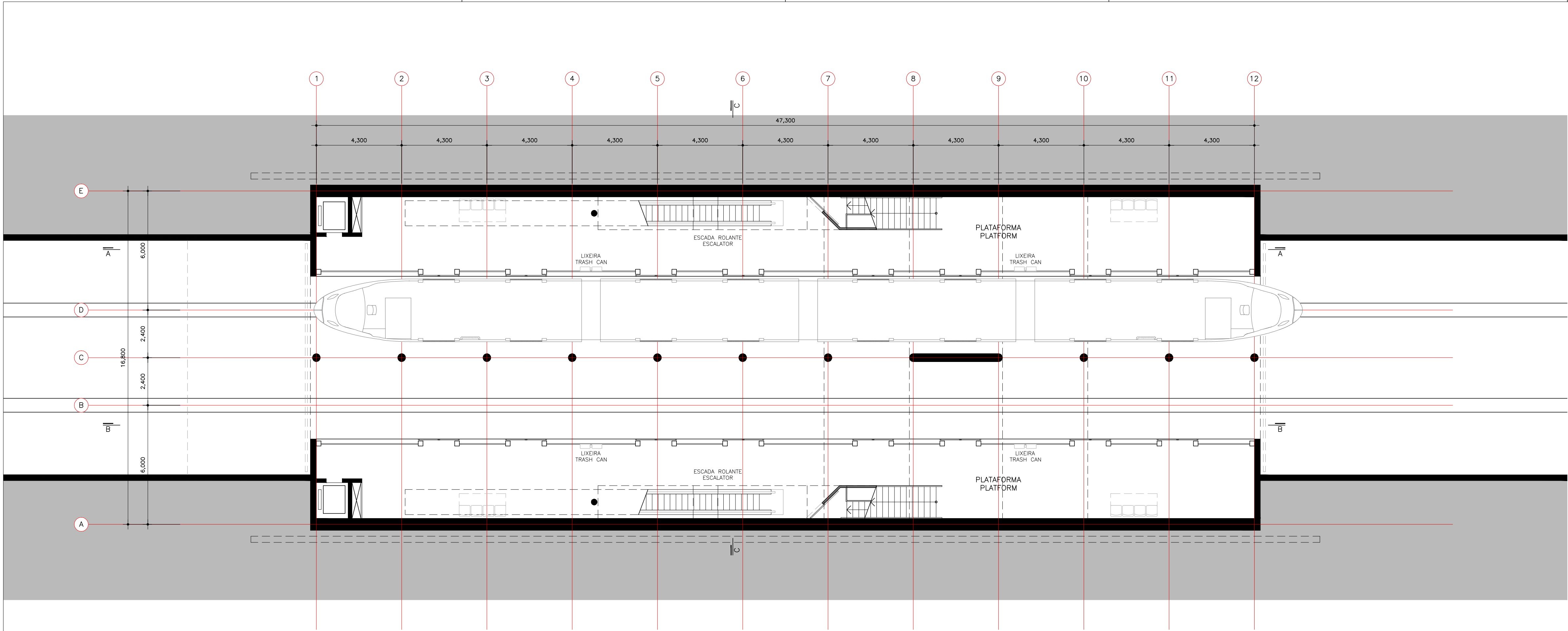
PLANTA NÍVEL 33.00 – PLATAFORMA | PLATFORM ESCALA | SCALE 1:125
