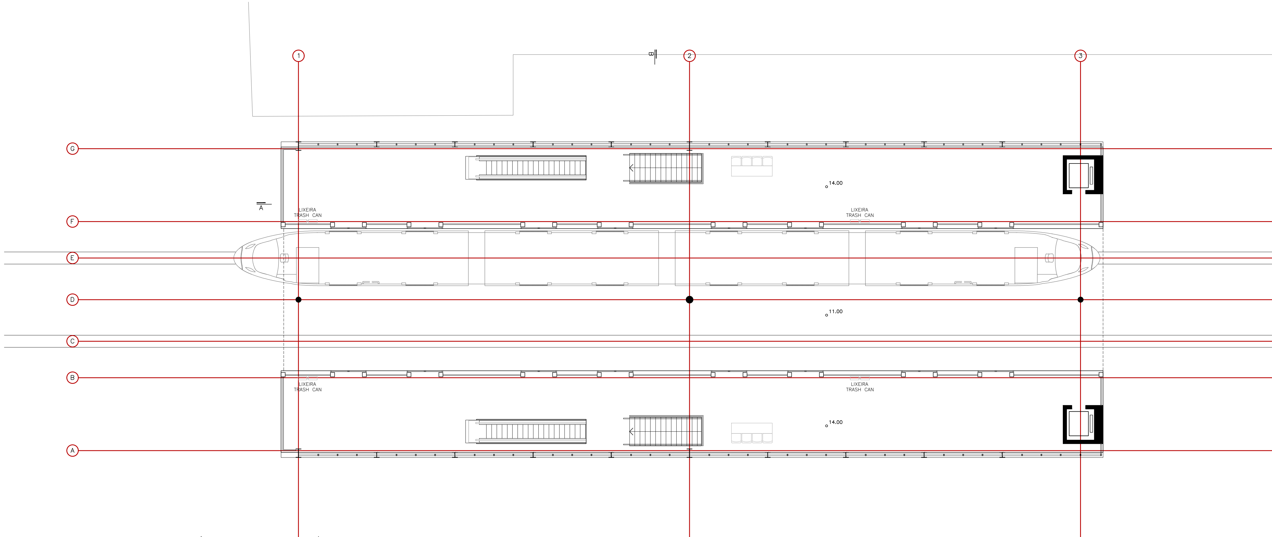
PLANTA NÍVEL 14.00 - PLATAFORMA | PLATFORM ESCALA | SCALE 1:125
