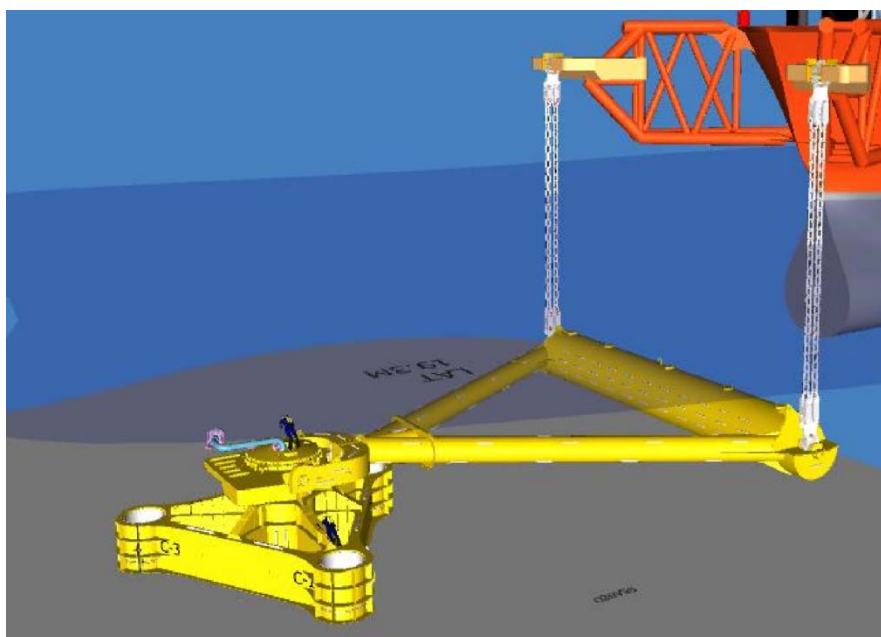
Figura 5-3: Arranjo típico do sistema submarino (o riser não está representado)
