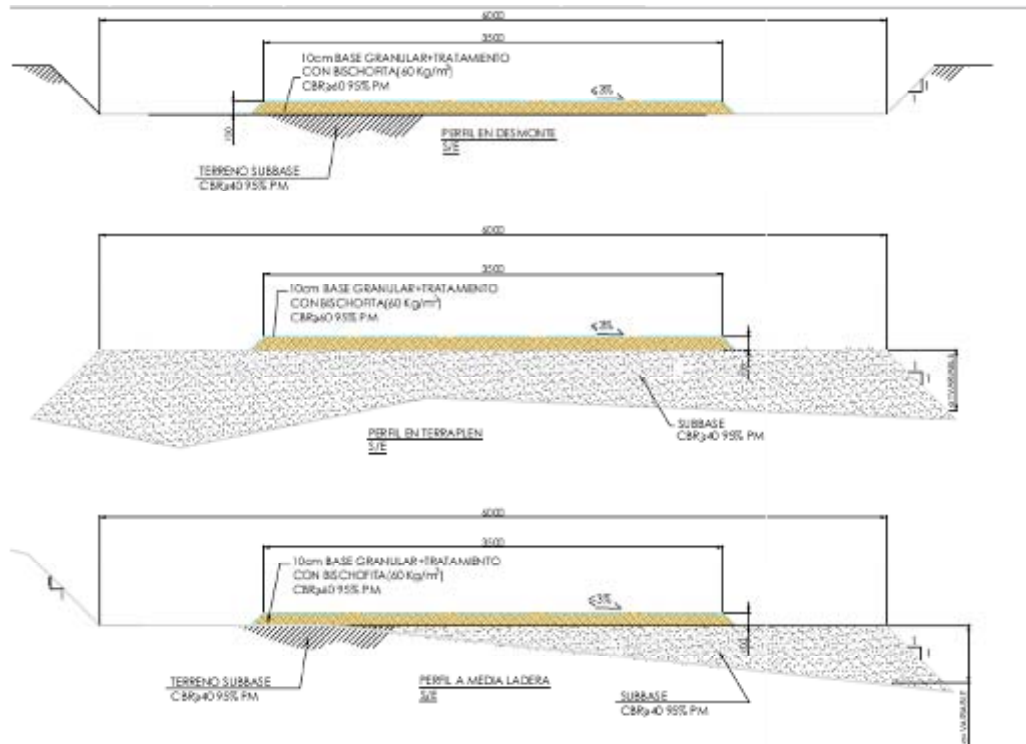
Figura 2.11 Perfil tipo de las áreas de maniobra de maquinaria y equipo del Proyecto.
