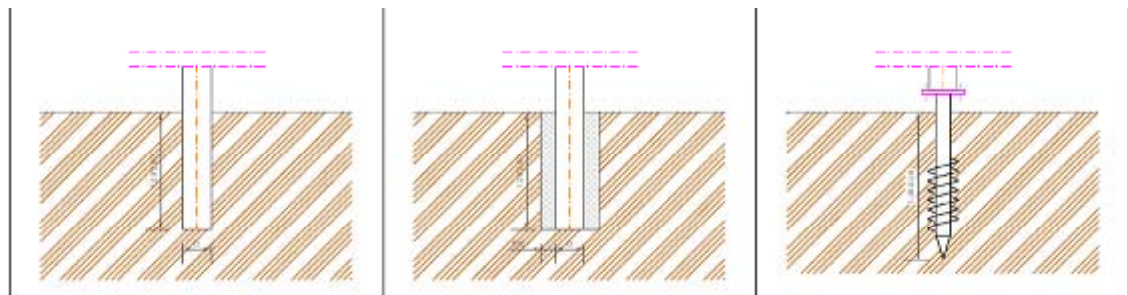
Figura 2.4 Estructura de soporte móvil típica de los módulos fotovoltaicos que se utilizarán para el Proyecto.
