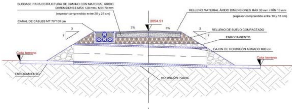
Figura 2.13 Sección típica de cruce.
