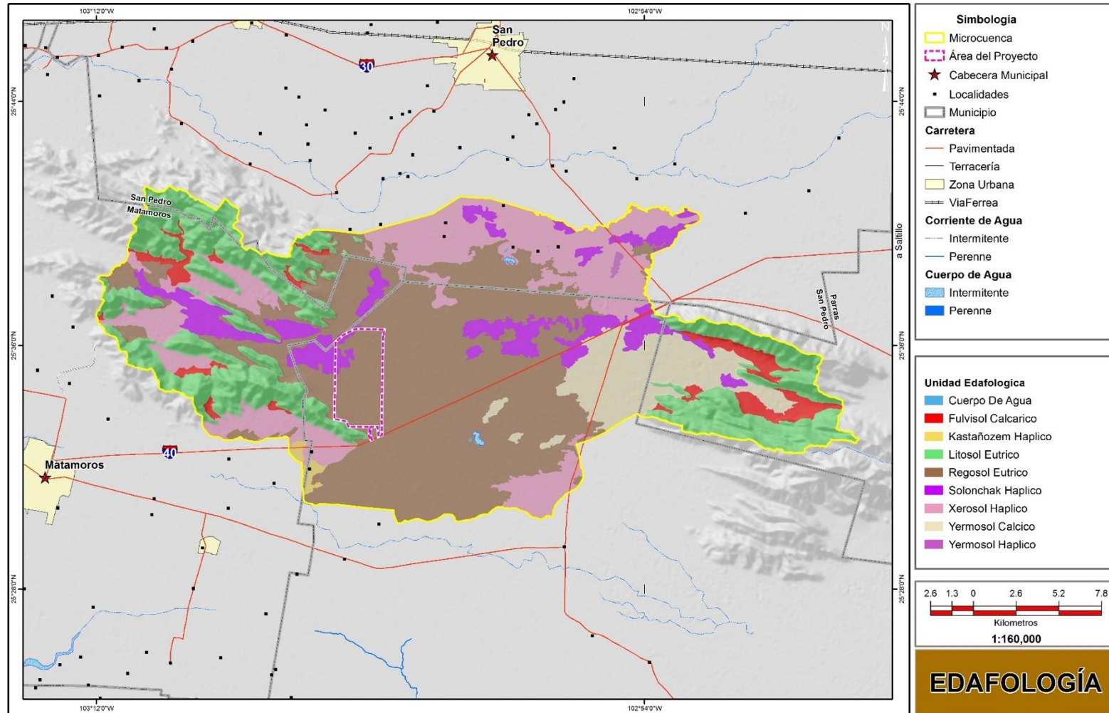
Figura 4.9. Edafología en el Sistema Ambiental y el Sitio del Proyecto Villanueva Solar.
