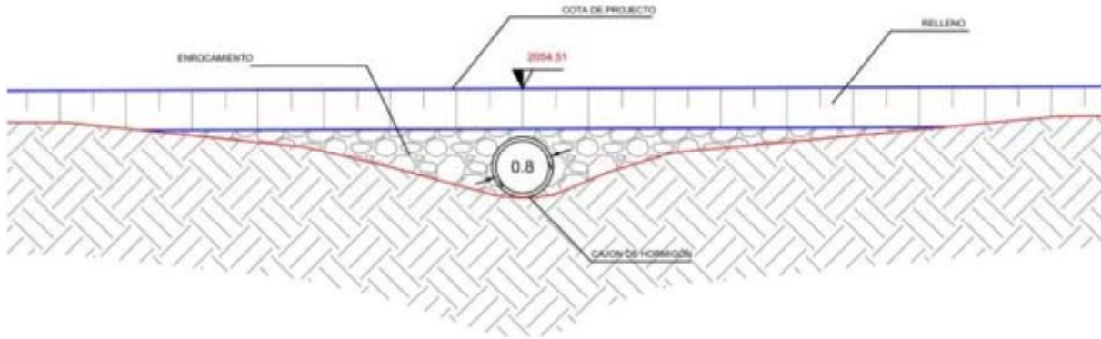
Figura 2.12 Perfil típico de cruce.
