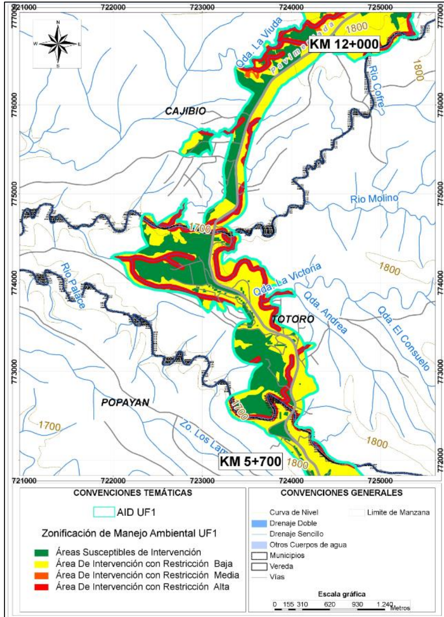
Figura 9.3 Zonificación de manejo ambiental K5+700-K12+000
