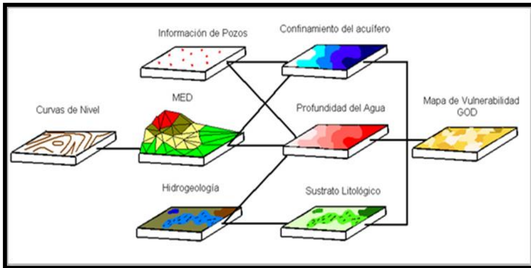
Figura 2.5 Método GOD. Fuente: Método de GOD, Foster. 1987.
