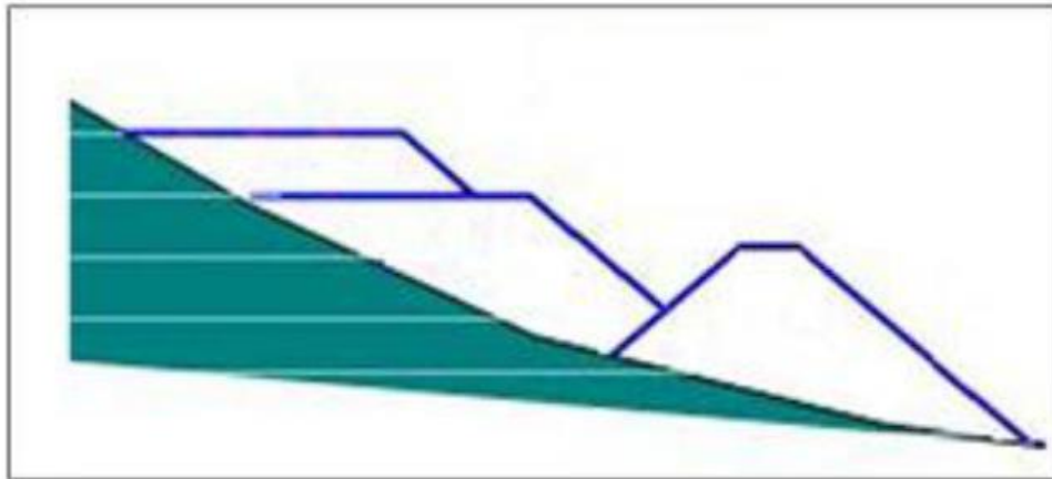
Figura 2.9 Diseño de ZODME en dique o muro de pie Fuente: Informe de diseño Fase II
