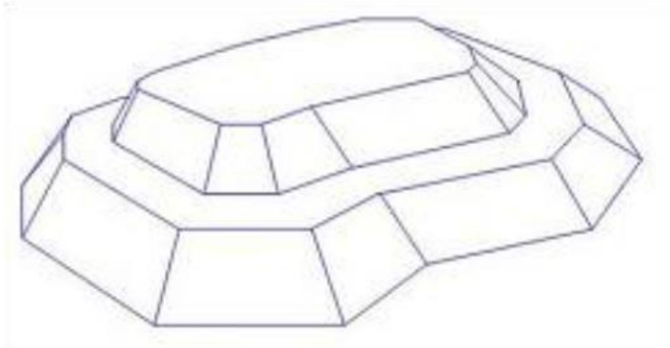
Figura 2.8 Diseño de ZODME en terraza
