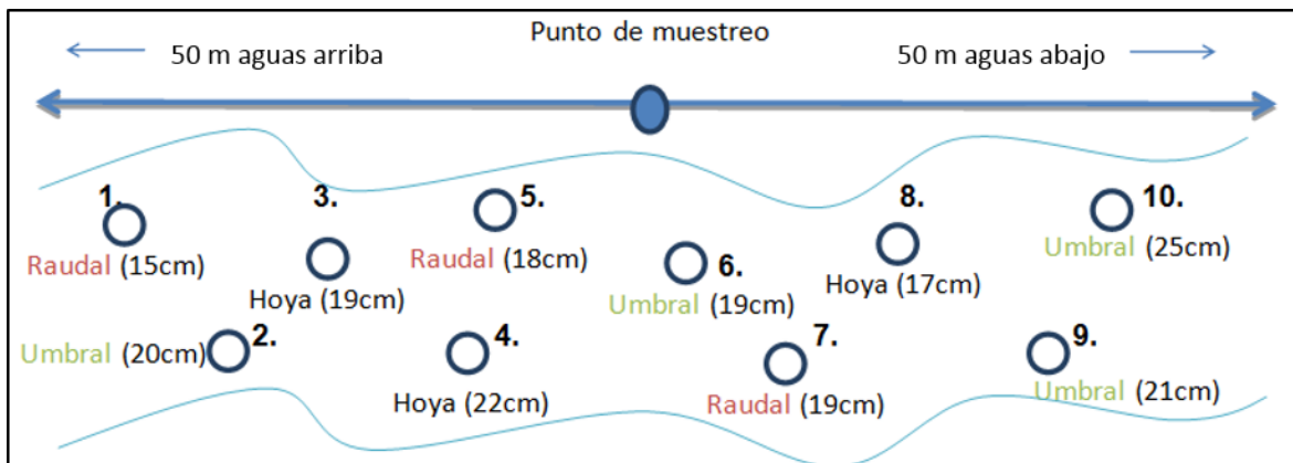
Figura 2.15. Esquema tipo para el monitoreo de comunidades bentónicas.
