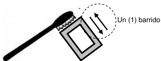
Figura 2.16. Forma correcta de realizar los raspados (barridos) en sustratos para el muestreo de perifiton.
