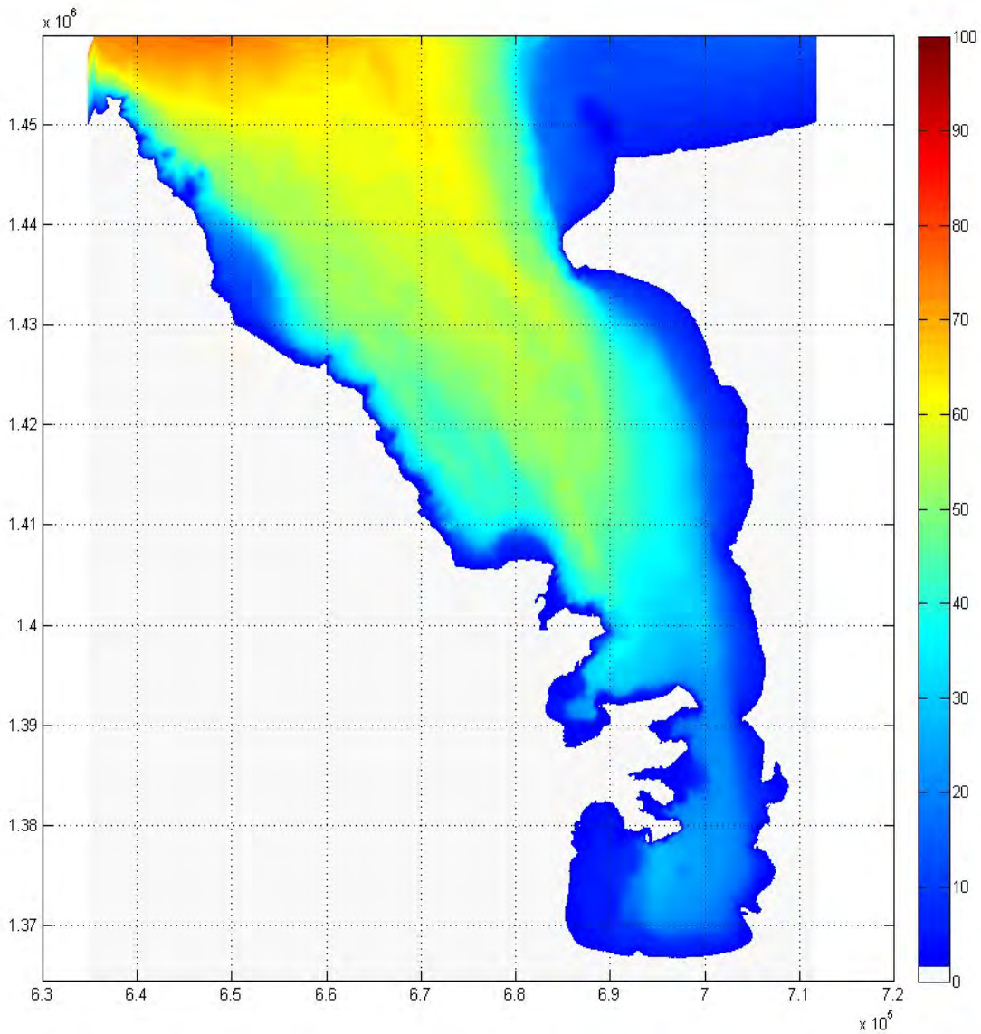
Figure Num. 3.46. Bathymetry of the Golfo de Urabá Source: Aqua&Terra Consultores Asociados S.A.S, 2015.
