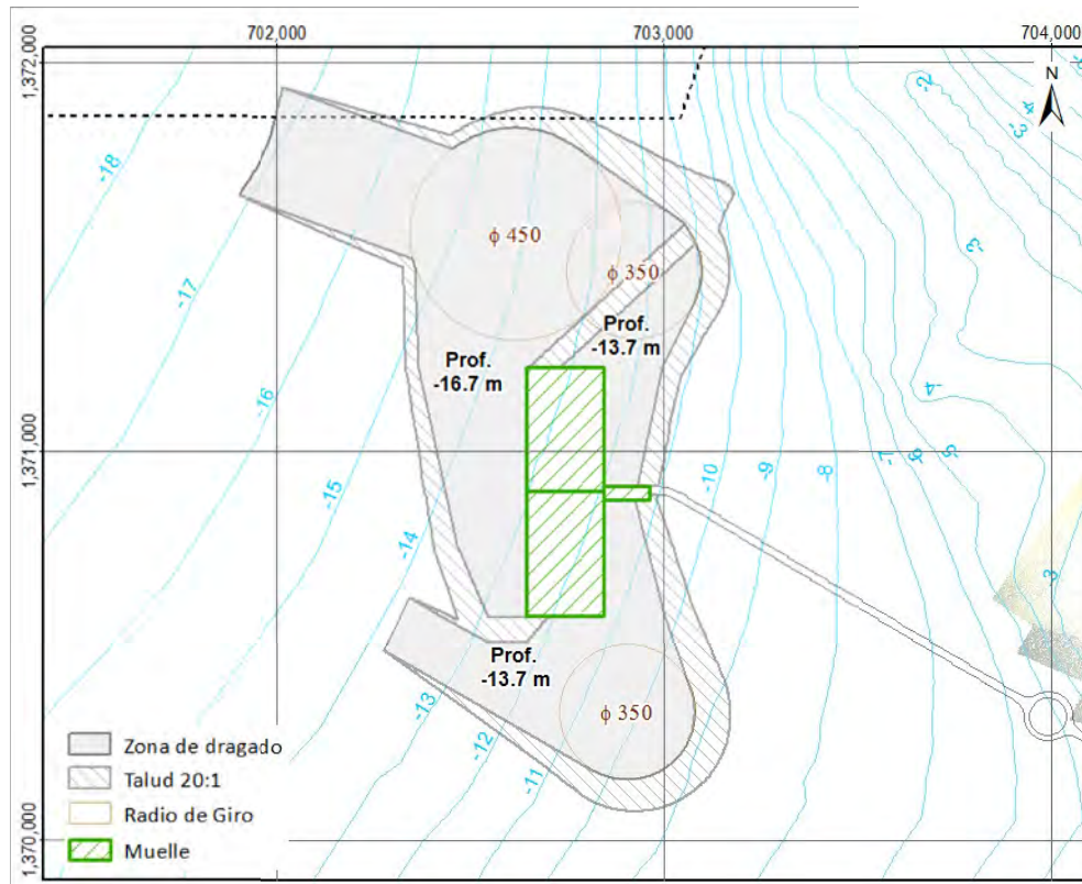
Figure Num. 3.16. Dredging areas. Source: Aqua & Terra Consultores SAS.
